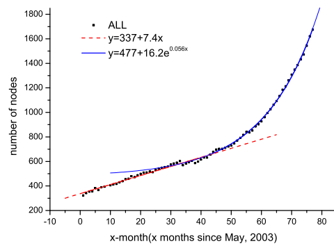
(d) Curve fittings for IPv6 (ALL)
