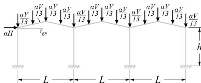
p) Frame case 16
