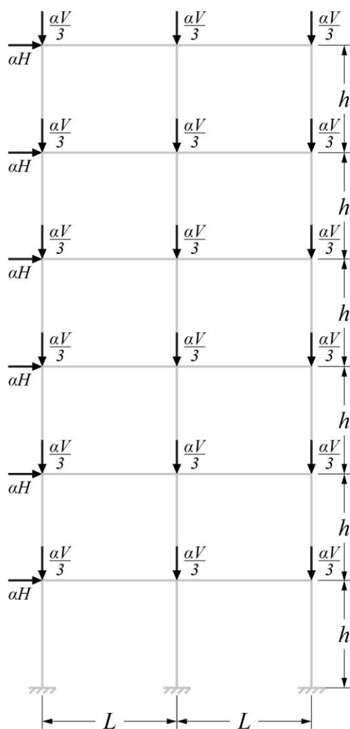
q) Frame case 17
